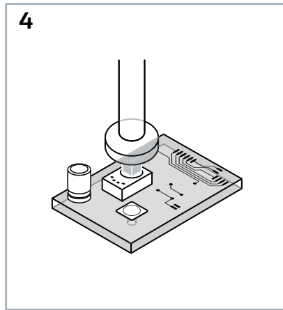
4 将MEMS芯片置于防护透气声学产品上
