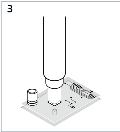
3 将防护透气声学产品置于PCB上
